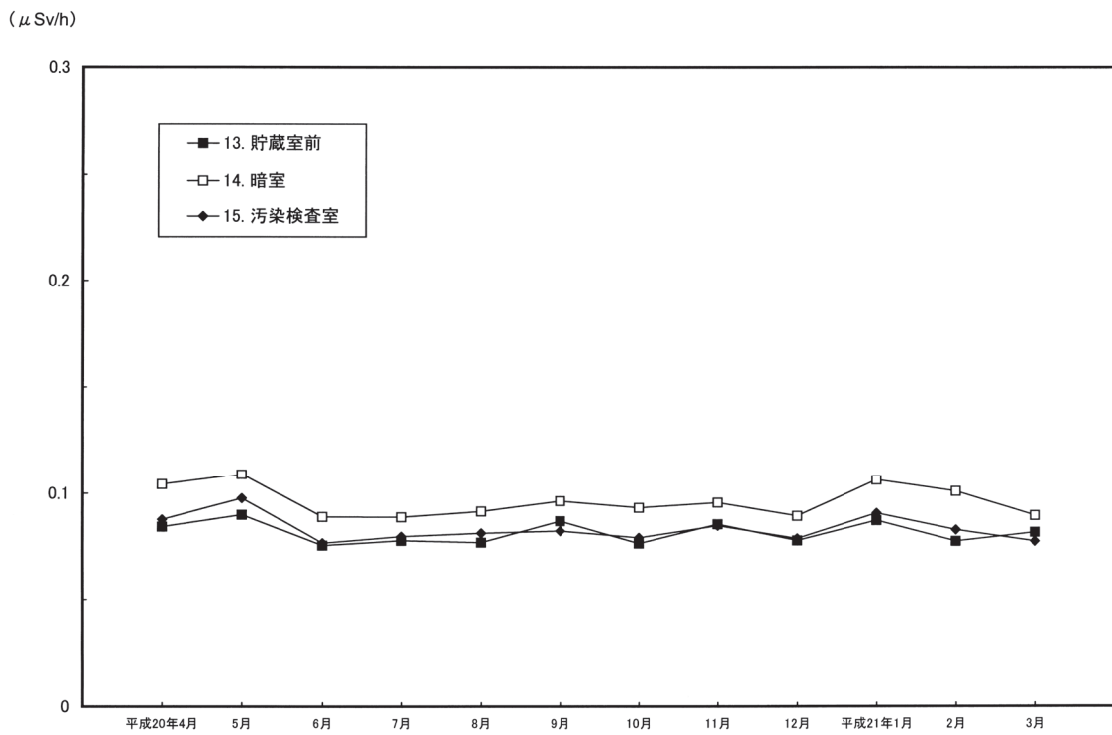
第 4-3 図 トレーサー・加速器棟における月間平均γ線量率の変動
