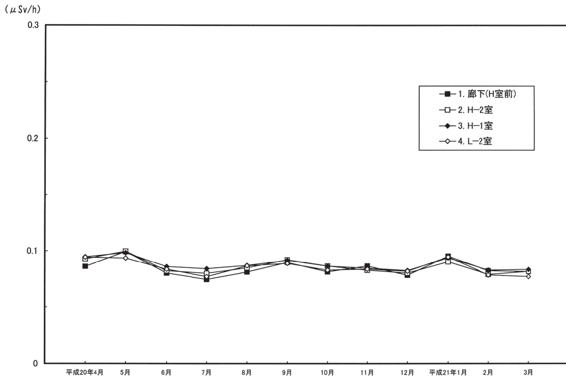
第 4-1 図 トレーサー・加速器棟における月間平均 \gamma 線量率の変動
