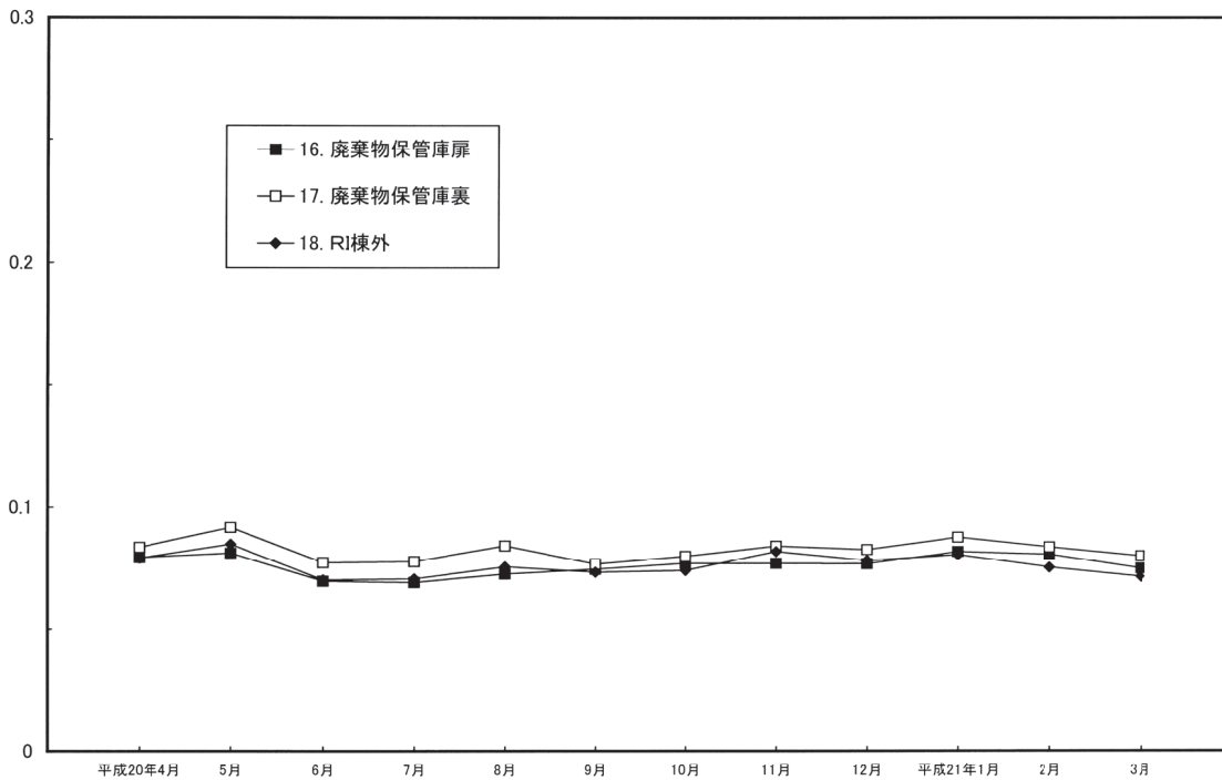
第 4-5 図 トレーサー・加速器棟における月間平均γ線量率の変動
