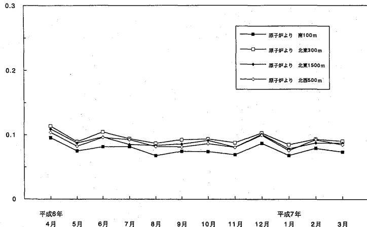
第8-2図 周辺監視区域境界における月間平均 \gamma 線線量当量率の変動
