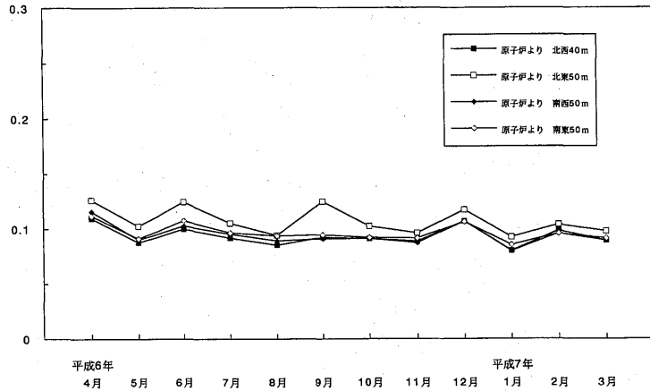
第8-1図 周辺監視区域境界における月間平均 \gamma 線線量当量率の変動 ( \mu\text{Sv/h} )
