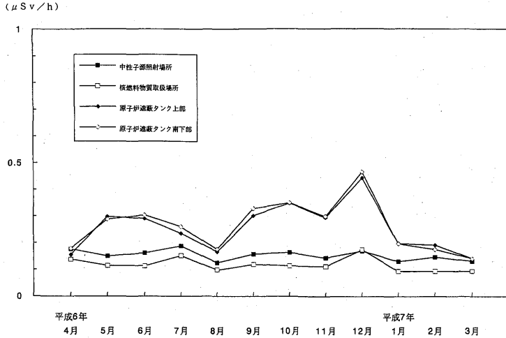
第2-2図 原子炉施設内における月間平均γ線線量当量率の変動
