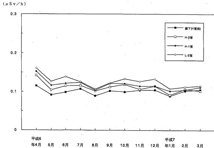
第4-1図 トレーサー・加速器棟内における月間平均 \gamma 線線量当量率の変動
