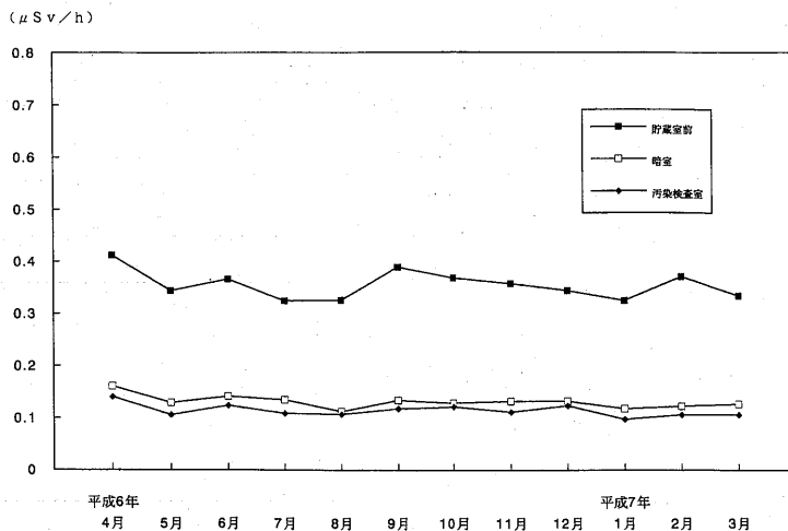
第 4-4 図 トレーサー・加速器棟内における月間平均 \gamma 線線量当量率の変動
