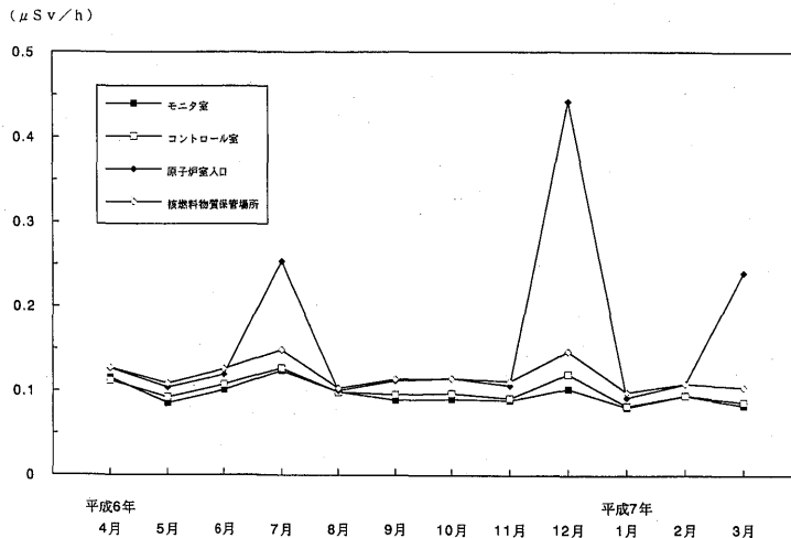
第2-1図 原子炉施設内における月間平均 \gamma 線線量当量率の変動
