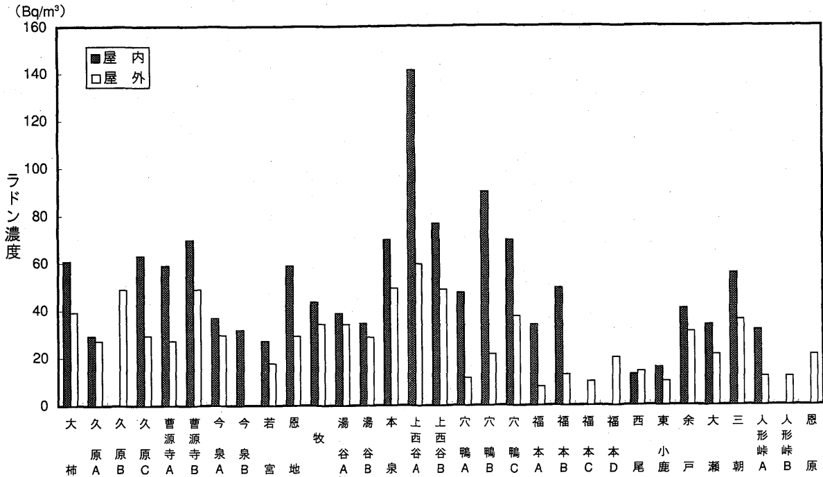
Fig. 7 三朝周辺地域における空气中ラドン濃度
