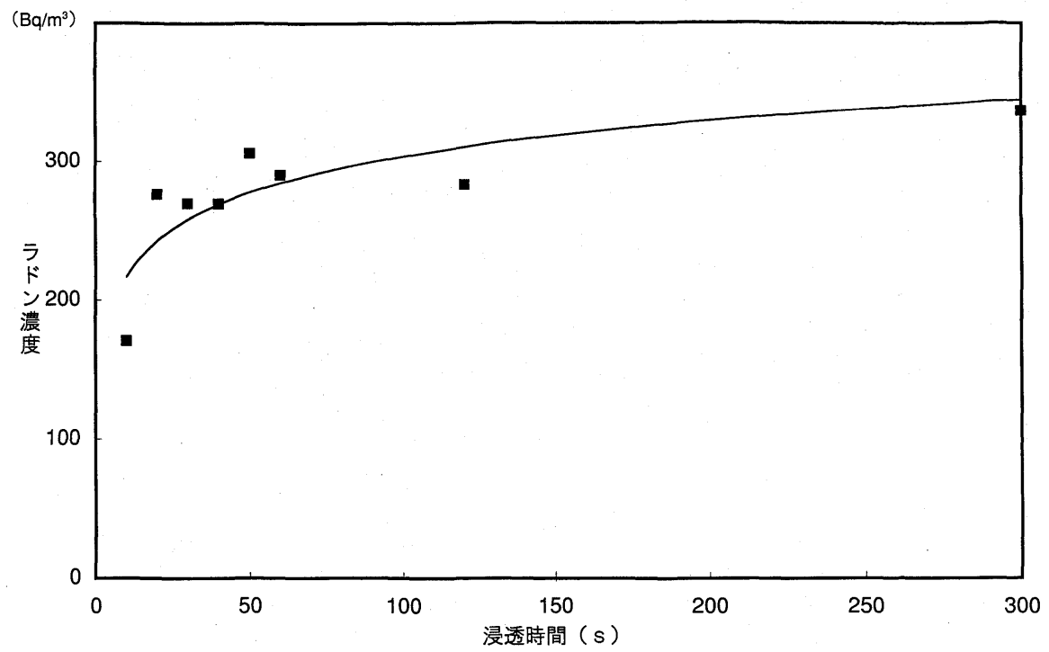
Fig. 5 浸透時間による溶出状況の変動
