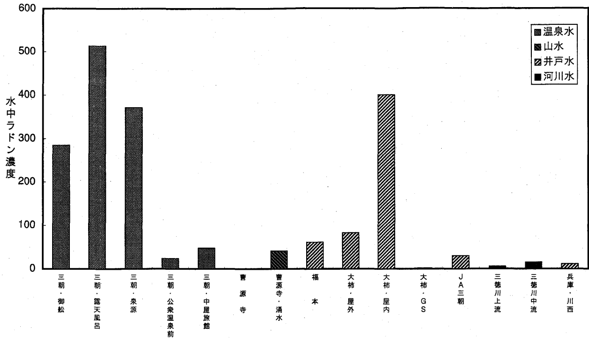
Fig. 9 三朝周辺地域における水中ラドン濃度
