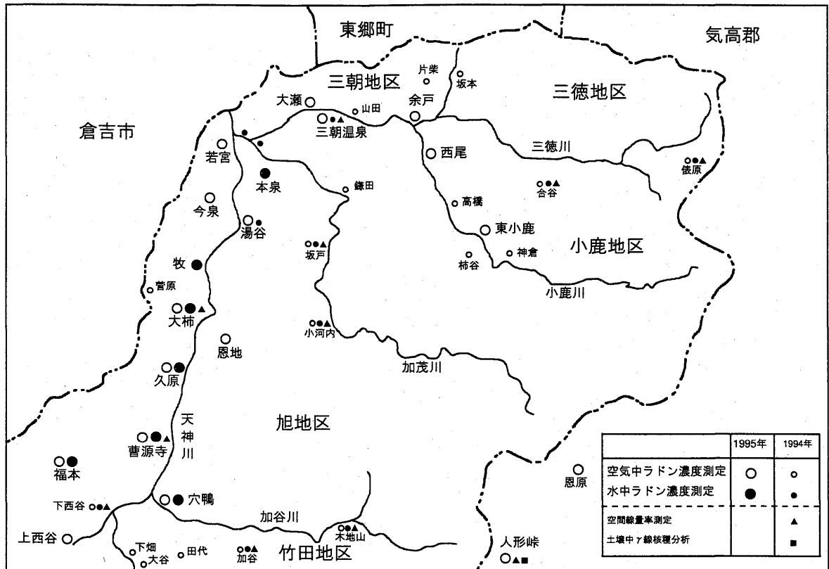
Fig. 1 三朝周辺地域における測定場所
