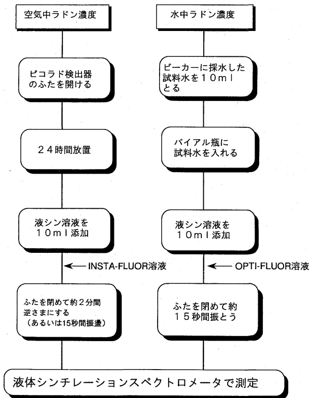
Fig. 2 ラドン濃度測定法
