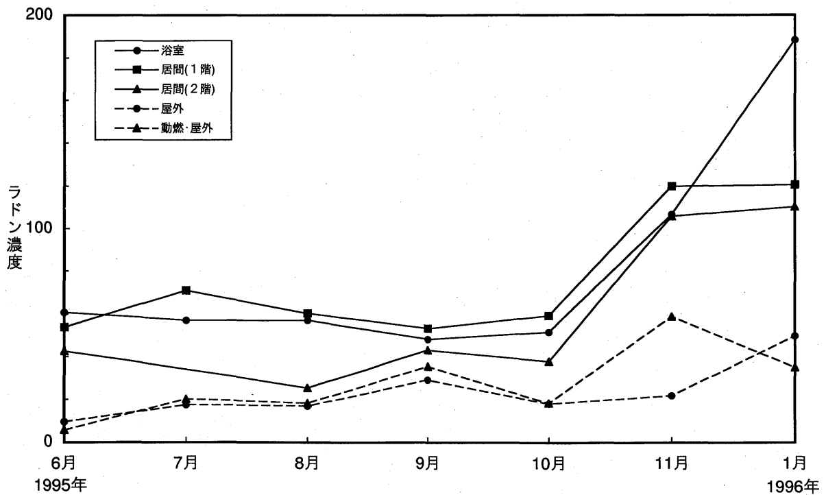
Fig. 10 三朝地域における空气中ラドン濃度の経時変化
