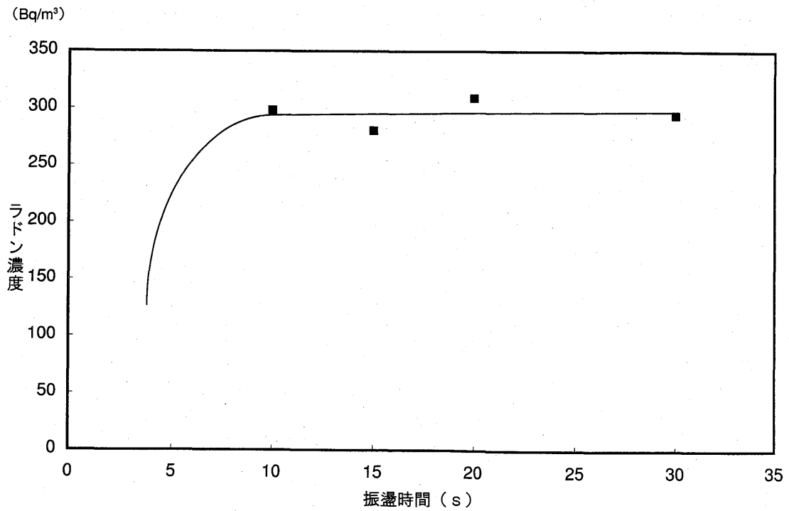
Fig. 4 振盪時間による溶出状況の変動
