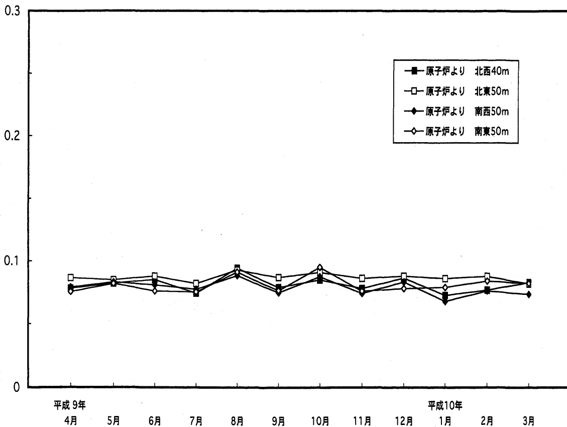
第 8 - 1 図 周辺監視区域境界における月間平均 \gamma 線線量当量率の変動
