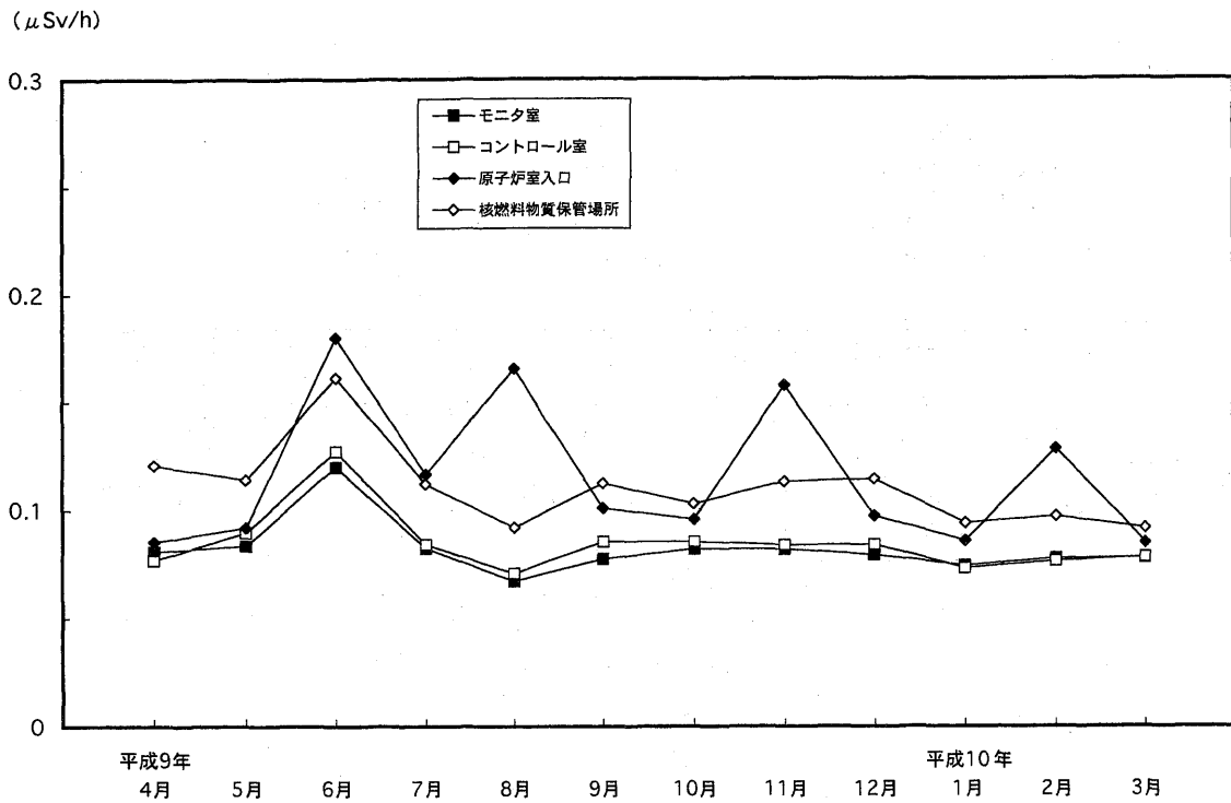
第 2 - 1 図 原子炉施設内における月間平均 \gamma 線線量当量率の変動
