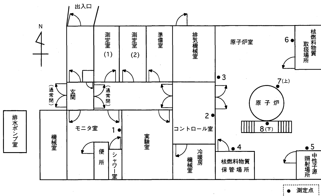
第 1 図 原子炉施設における \gamma 線線量当量率測定点
