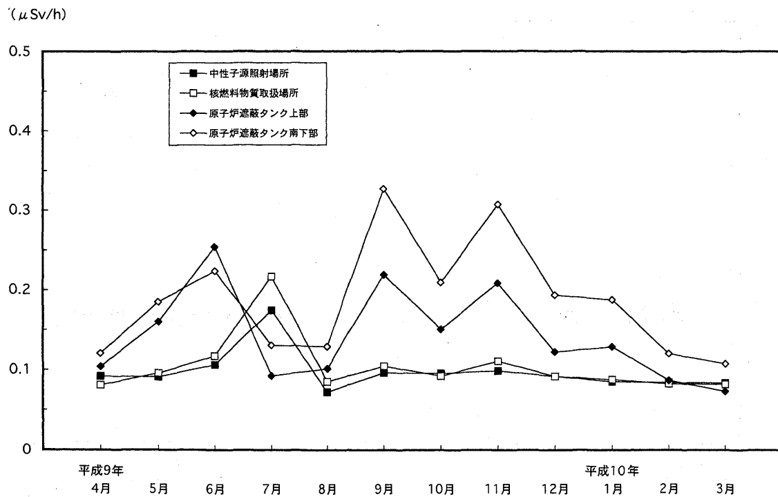
第 2 - 2 図 原子炉施設内における月間平均 \gamma 線線量当量率の変動
