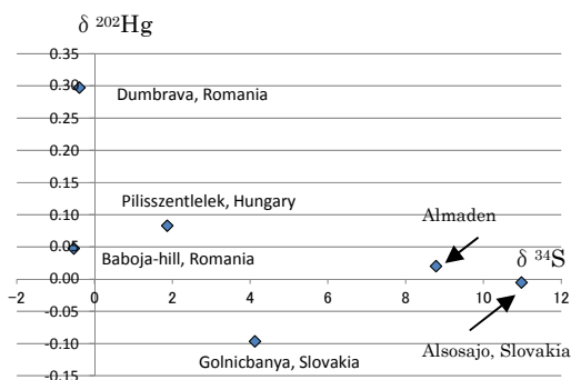
図 1. ヨーロッパの辰砂鉱山鉱石の硫黄同位体比と水銀同位体比の二次元グラフ
