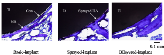
図 3 イヌ脛骨にインプラントした HA 被覆人工歯根の骨伝導状態
