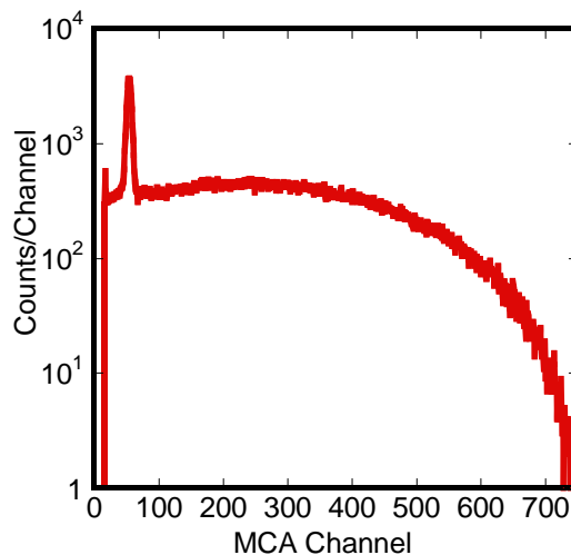
図 1 CsI シンチレータの放射化によって得られたエネルギースペクトルの例
