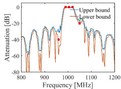
図 14 : SAW フィルタの通過特性
