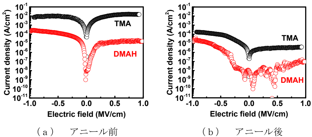
図3 Al_2O_3 /diamond MOSキャパシタのJ-E特性
