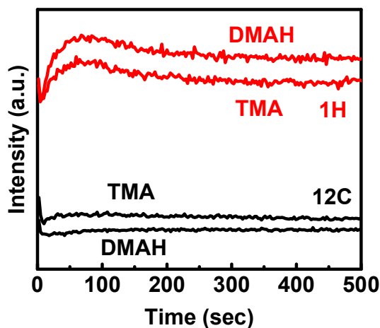
図1 SIMS 定量測定
