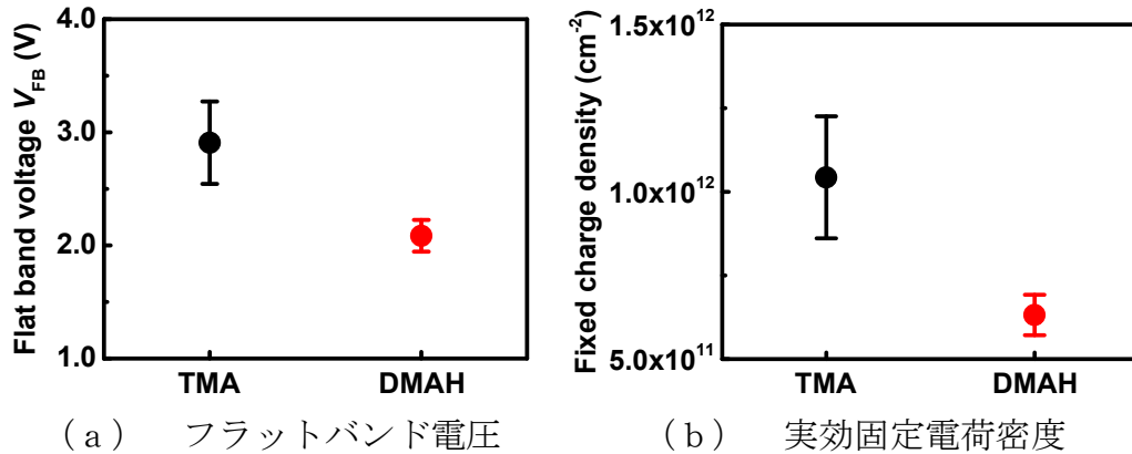
図2 C-V測定結果
