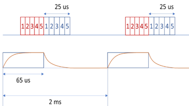
Fig. 2 パルス照明, 発光, 撮影パターン
