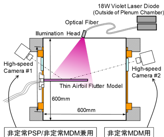
Fig. 3 JAXA における実験の概要
