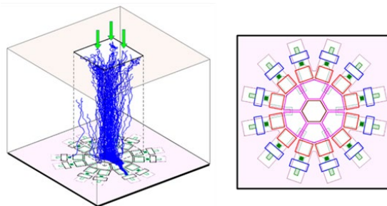
Fig. 8 ブランディングイメージセンサ「花火」立体的な信号電子の軌跡 (左)；表面側の電極配置 (右)
