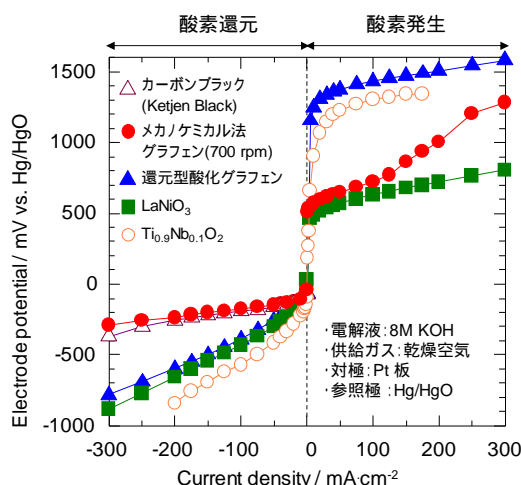
図3 メカノケミカル反応後のグラフェンとその他の材料の酸素還元・酸素発生活性の比較
