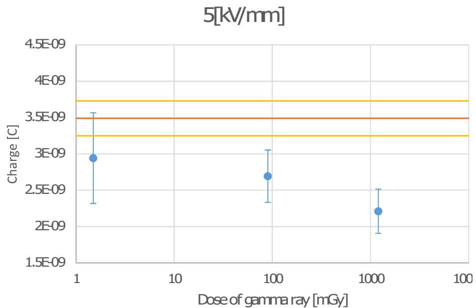
図 3. 未照射および照射 LDPE（照射 1 日後）の積分電荷特性
