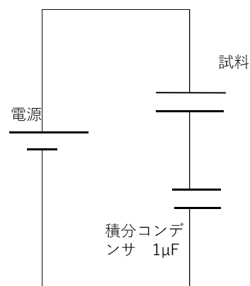
図 2. 電流積分電荷法の実験回路
