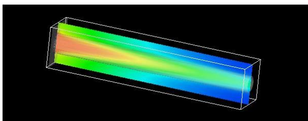
流体運動と固体熱伝導の一括解析の一例
