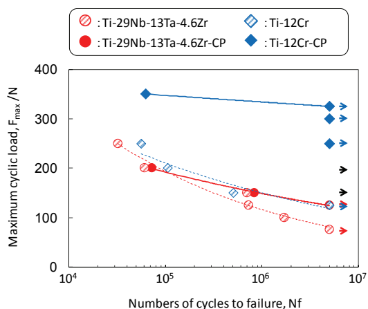
図6 Ti-12 合金製ロッドおよび Ti-29Nb-13Ta-4.6Zr 合金製ロッドを用いた脊椎固定器具の ASTM F1717 試験結果
