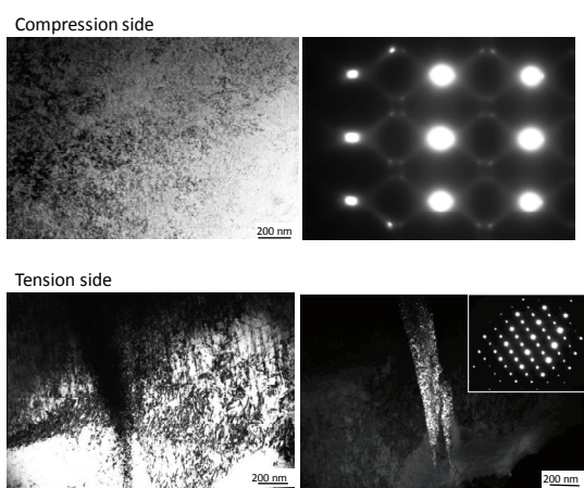
図3 曲げ変形後のTi-12Cr合金製ロッド断面の曲げ変形内側部（圧縮側）および外側部（引張側）のTEM観察結果
