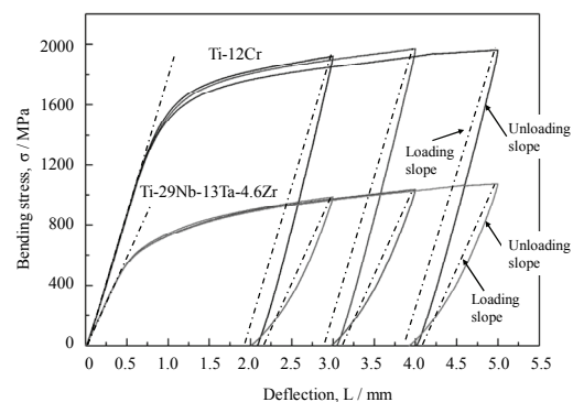
図4 Ti-12Cr合金製ロッドおよびTi-29Nb-13Ta-4.6Zr合金製ロッドの曲げ応力-変位曲線
