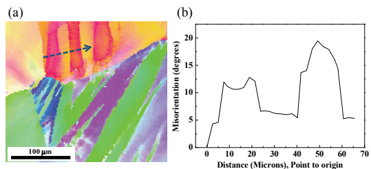
図 2 曲げ変形後の Ti-12Cr 合金製ロッド断面の曲げ変形外側部の EBSD 分析結果: (a) 結晶方位分布, (b) (a) 中の矢印上の結晶方位変化
