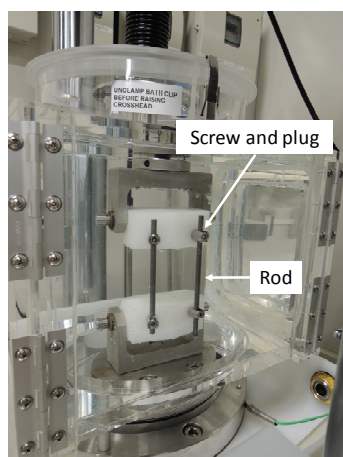
図5 ASTM F1717 試験のセットアップ写真
