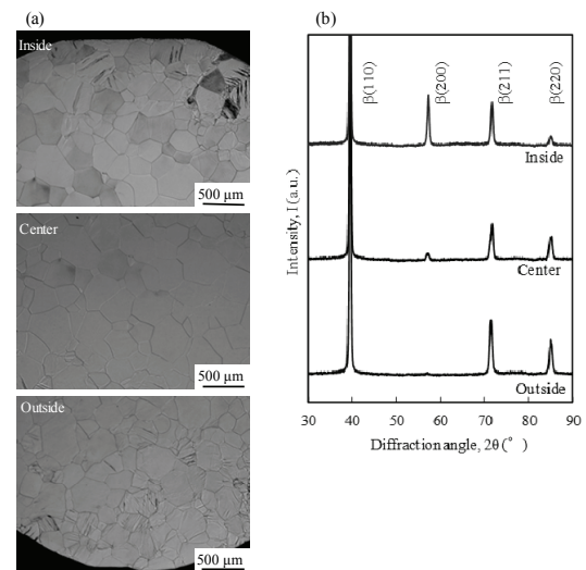
図 1 曲げ変形後の Ti-12Cr 合金製ロッド断面の曲げ変形内側部、中央部および外側部の (a) OM 観察結果および (b) XRD 分析結果
