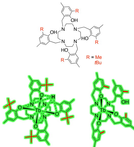
図1 「酸素応答性を有する強発光性のテルビウム錯体」における配位子の化学修飾による配位環境の制御 (R = tBu: 八配位, R = Me: 七配位)。
