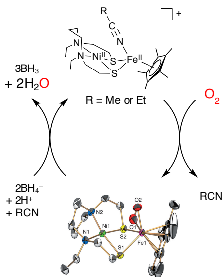
図3 ニッケル-鉄二核錯体を用いた酸素分子の水への還元反応(図中には、鍵となる活性酸素中間体であるペルオキシ化合物の結晶構造を示した)。
