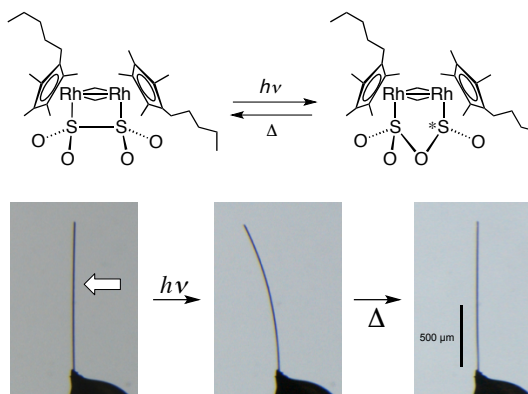
図2 光感応性のロジウム二核錯体とその針状結晶が示す可逆な光誘起屈曲現象。
