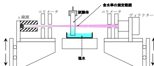
図1 ガンマ線を用いた塩溶液の浸透実験(材料内の塩濃度・塩の析出量に応じた水分伝導率を測定)
