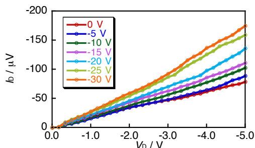
図8, CuBrBu微結晶を用いたFETの出力特性
