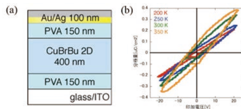
図6, 強誘電体キャパシタとヒステリシス曲線
