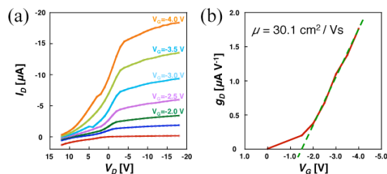
図4, 単結晶FETの出力特性(a)と伝達特性(b)
