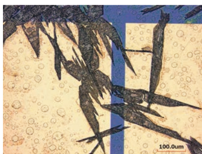
図7, 溶媒噴出法によって作製したCuBrBu微結晶
