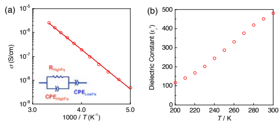
図3, (a)伝導度および(b)誘電率の温度依存性
