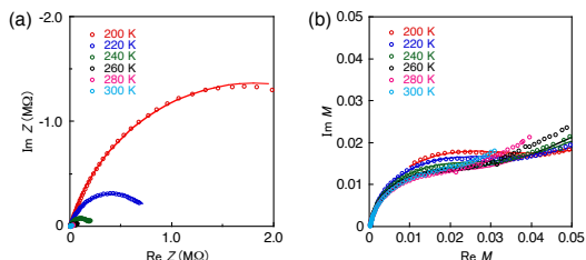
図2, (a) Zおよび(b) MのCole-Coleプロット
