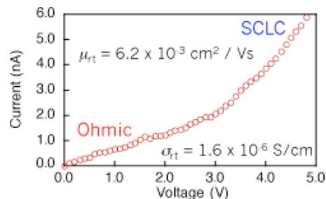
図5, 強誘電性配位高分子薄膜のI-V特性
