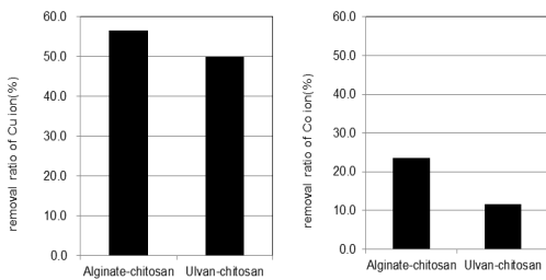
図．ウルバン - キトサンゲルおよびアルギン酸 - キトサンゲルの重金属イオン吸着能力比較
