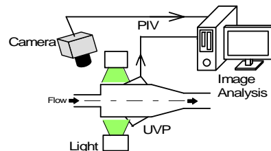
図3. 分散制御法試験装置図
