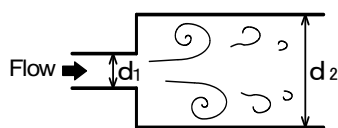
図2. 高濃度パルプ繊維の分散を可能にする急拡大流路
