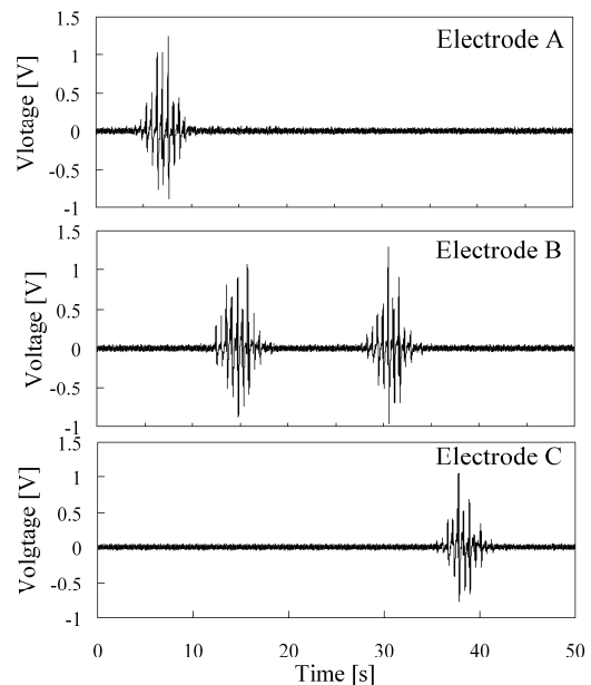
図 4 歩行信号波形
