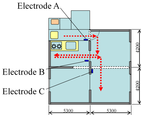
図 1 電極配置場所と室内歩行経路
